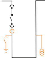
Vakum kesicili kuplaj ve bara yükseltme panosu
